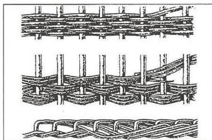
Différents types de clayage
